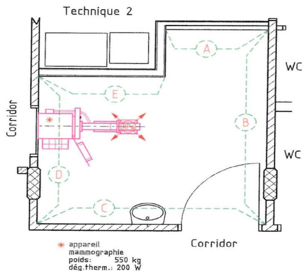
Abbildung 14: Beispiel eines Strahlenschutzplans für eines Mammographie-Roentgensystems
