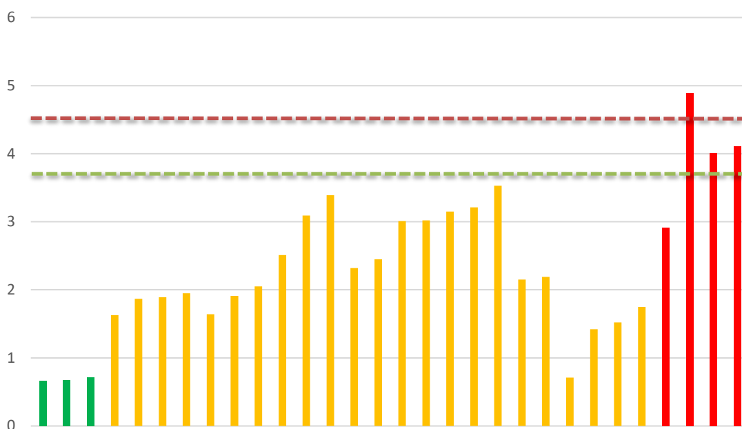
Abbildung 34: Dosen in mGy für eine Brustdicke von 75 mm, gemessen in einer Stichprobe von 30 unterschiedlichen Systemen verschiedener Hersteller
