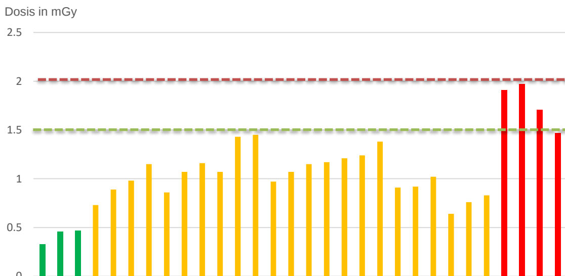
Abbildung 33: Dosen in mGy für eine Brustdicke von 45 mm, gemessen in einer Stichprobe von 30 unterschiedlichen Systemen verschiedener Hersteller
