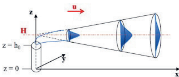
Figura A3-1: rappresentazione schematica dei parametri utilizzati per i calcoli della propagazione.
